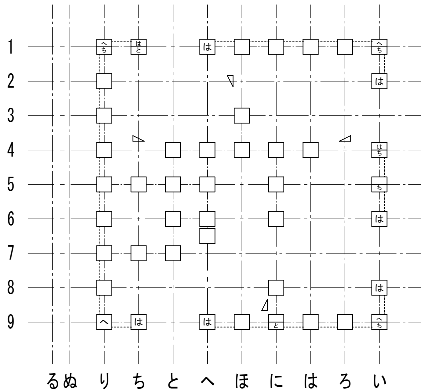
2階柱壁伏図
