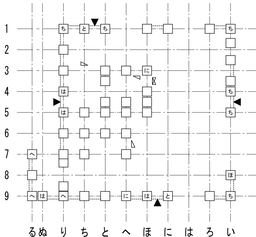
1階柱壁伏図
